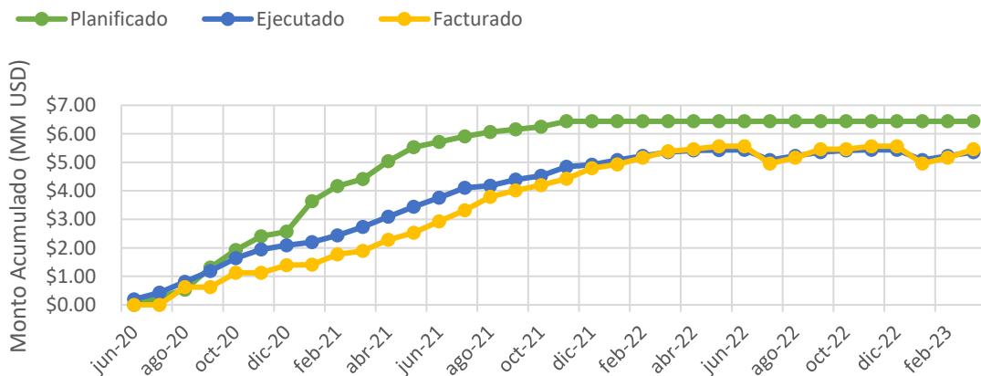
Curva S - Lote 7 NAGU102
